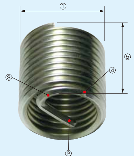
各部の名称
