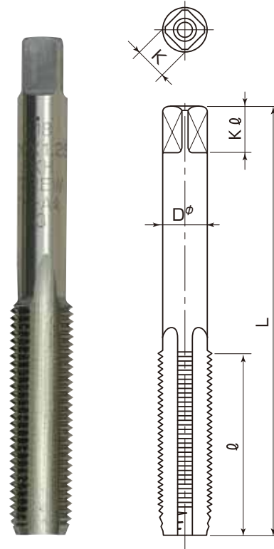
#3上タップ(食付き1.5山)
