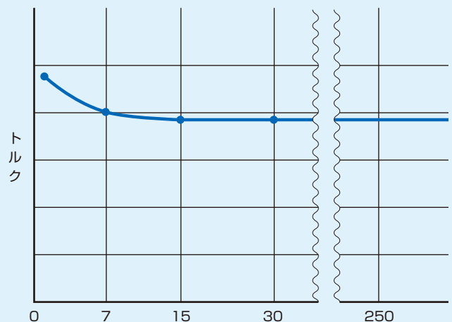
ロックタイプスプリュートルク性能曲線
